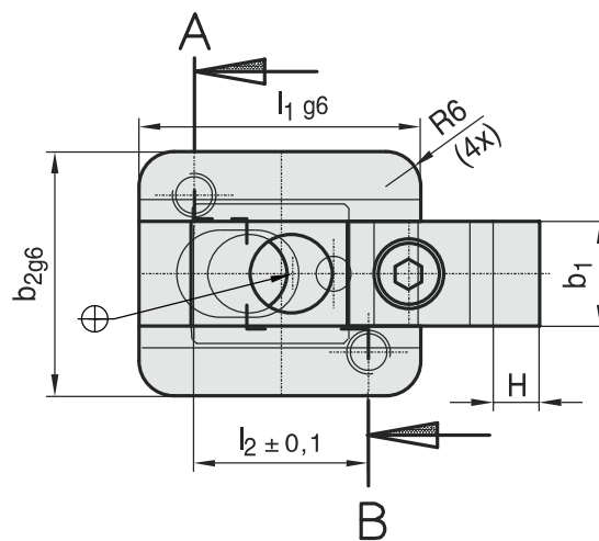
Шариковый стопор с пружиной AC-AZ374...
