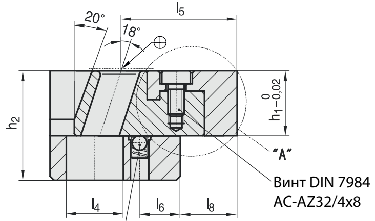
Шариковый стопор с пружиной AC-AZ374...
